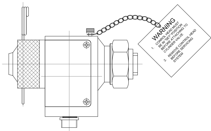
R.H.SIDE VIEW
